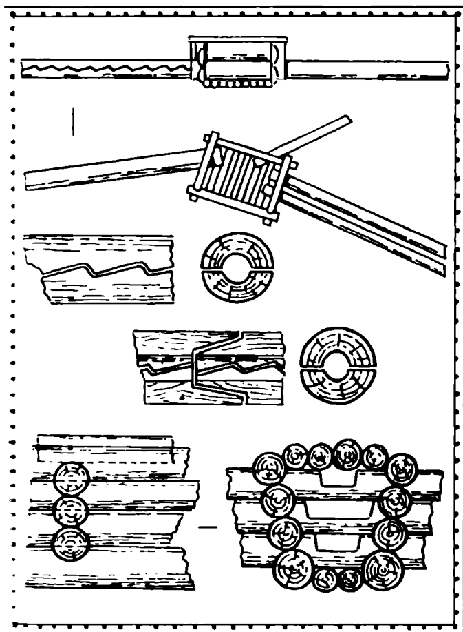
Детали древнерусских водоотводных сооружений
